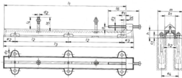
Ausführung C Nennlänge l_1 = 1600 bis 2200 mm
