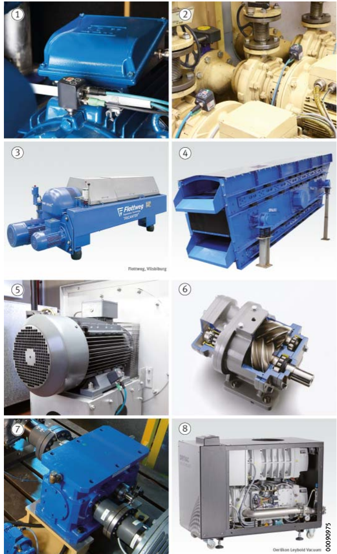
Bild 3 Überwachte Aggregate
