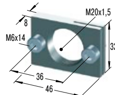
RF20 Rechteckflansch
