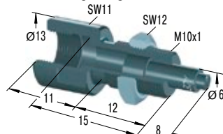
BV10SC Bolzenvorlagerung
