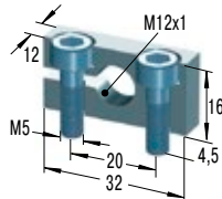
MB12 Klemmflansch
