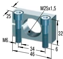
MB25 Klemmflansch
