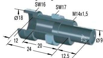
BV14 Bolzenvorlagerung
