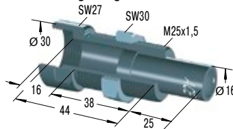
BV25SC Bolzenvorlagerung
