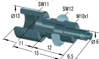
BV10 Bolzenvorlagerung
