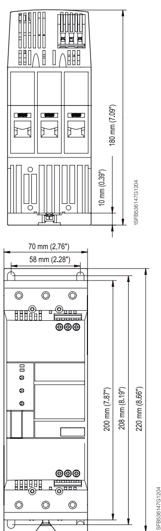
PSR60 ... 105 PSRC60 ... 105
