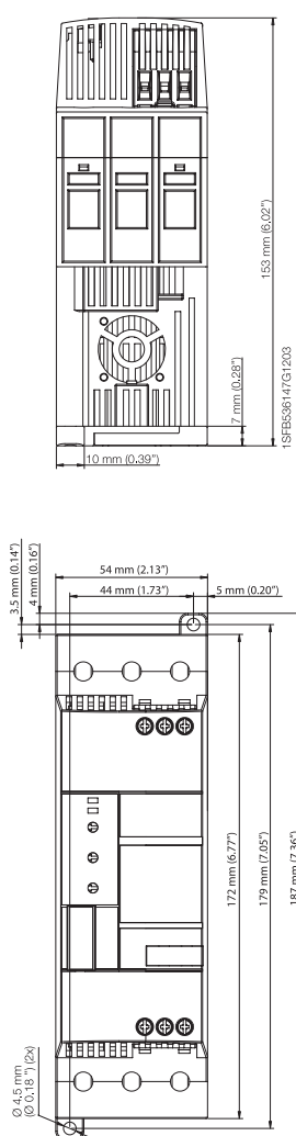
PSR37 ... 45 PSRC37 ... 45
