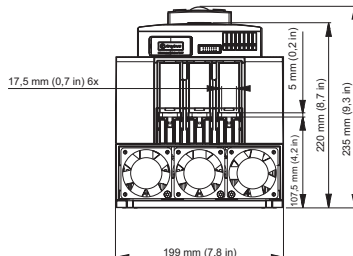
PSTX142 ... PSTX170
