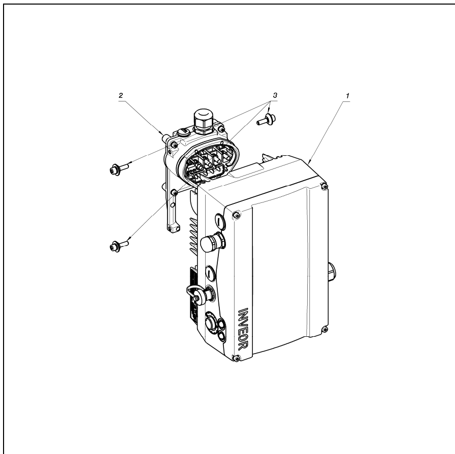
Abb. 14: Antriebsregler aufsetzen
