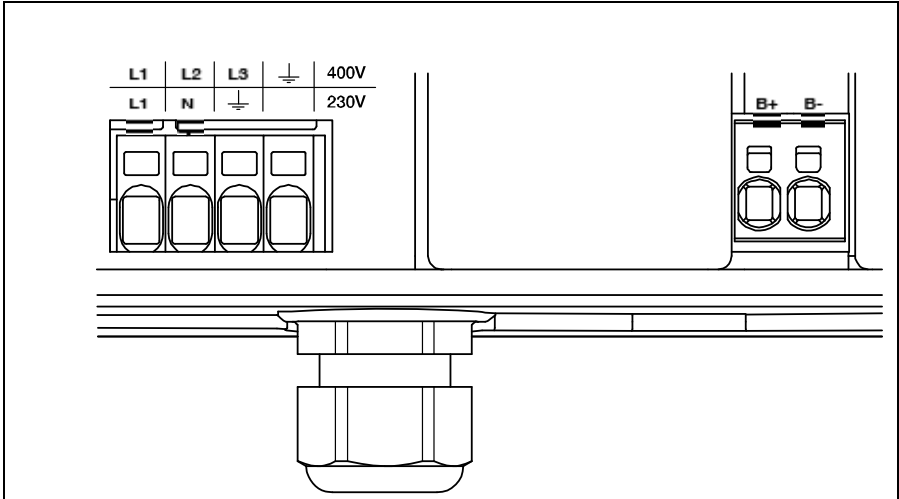
Abb. 7: Leistungsanschluss
