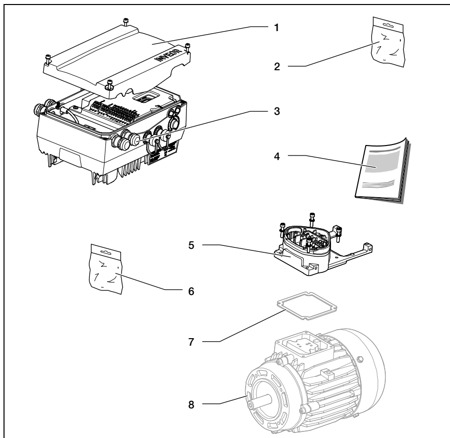
Abb. 2: Lieferumfang
