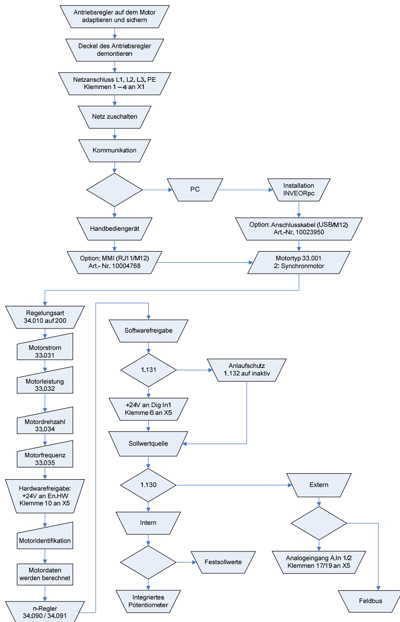
Abb. 28: Blockdiagramm Schnellinbetriebnahme SM
