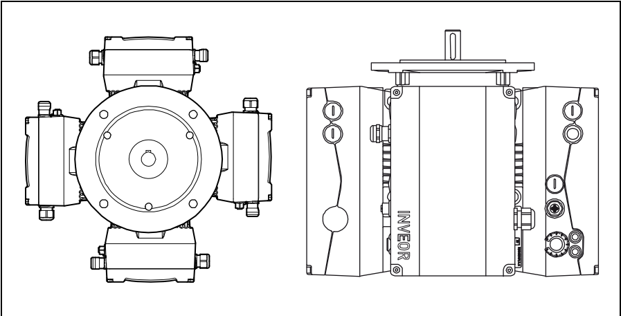
Abb. 3: Motoreinbaulage/Zulässige Ausrichtungen
