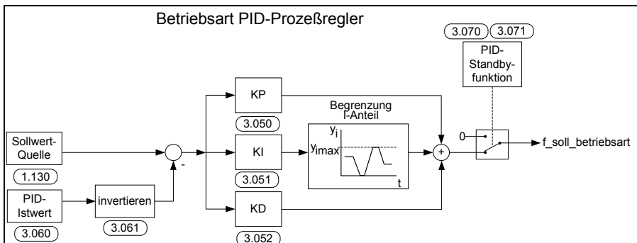
Abb. 18: PID-Prozessregelung
