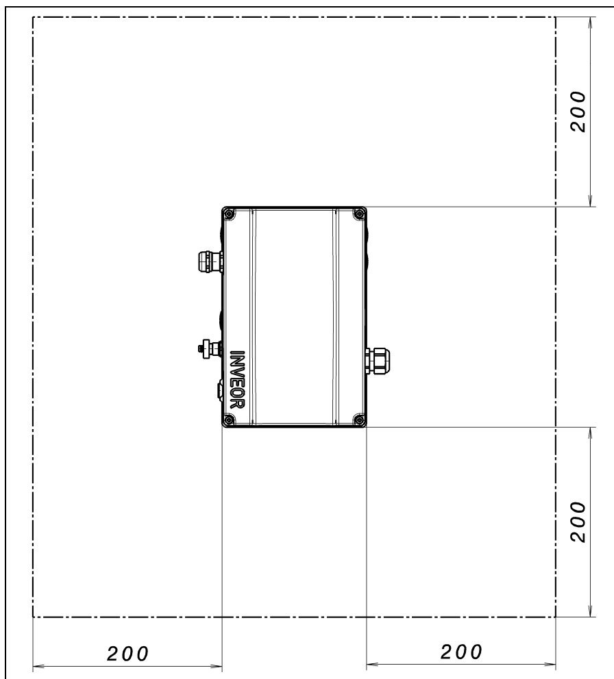
Abb. 10: Mindestabstände
