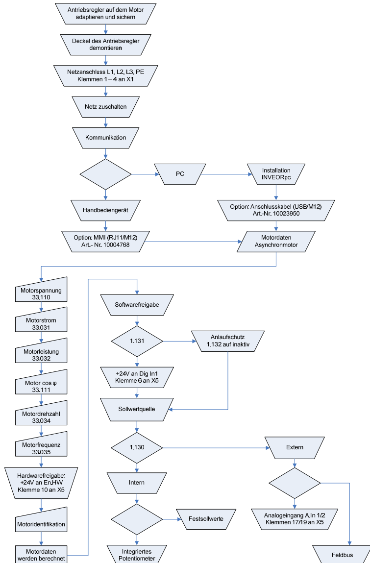
Abb. 27: Blockdiagramm Schnellenbetriebnahme ASM
