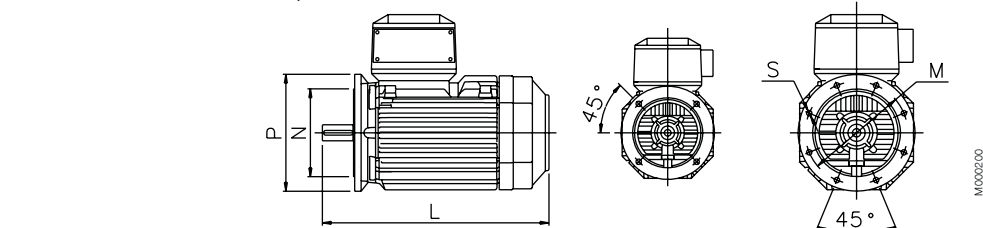
Flange-mounted motor IM 3001, IM B5
